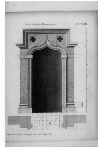
Abb. 65 und 66 Gotische Mustervorlagen aus Batty Langleys „Gothic Architecture...“
