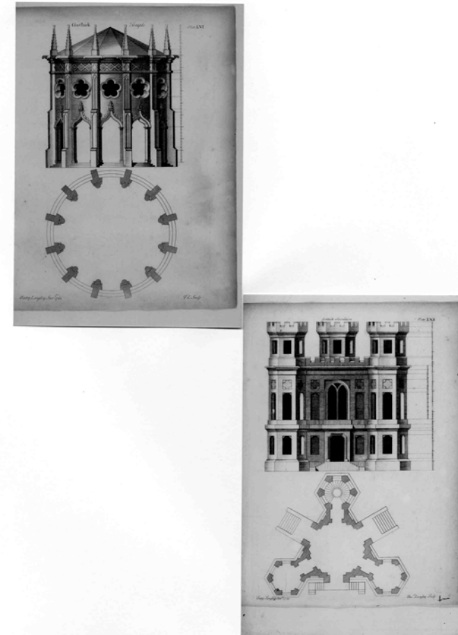
Abb. 69 und 70 Vorlagen für gotische Tempel und Pavillons aus Batty Langleys „Gothic Architecture ...“
