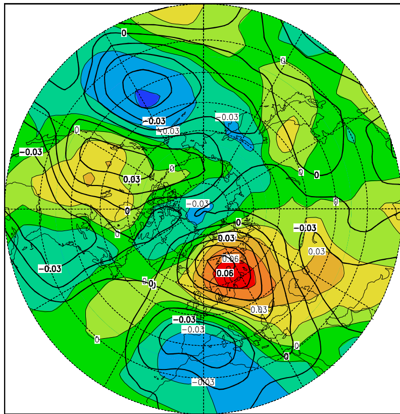
Abbildung A82: 7. Eigenvektor des Dezembers (4,7%)
