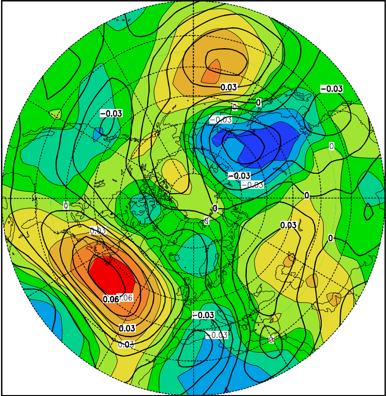
Abbildung A81: 6. Eigenvektor des Dezembers (5,5%)
