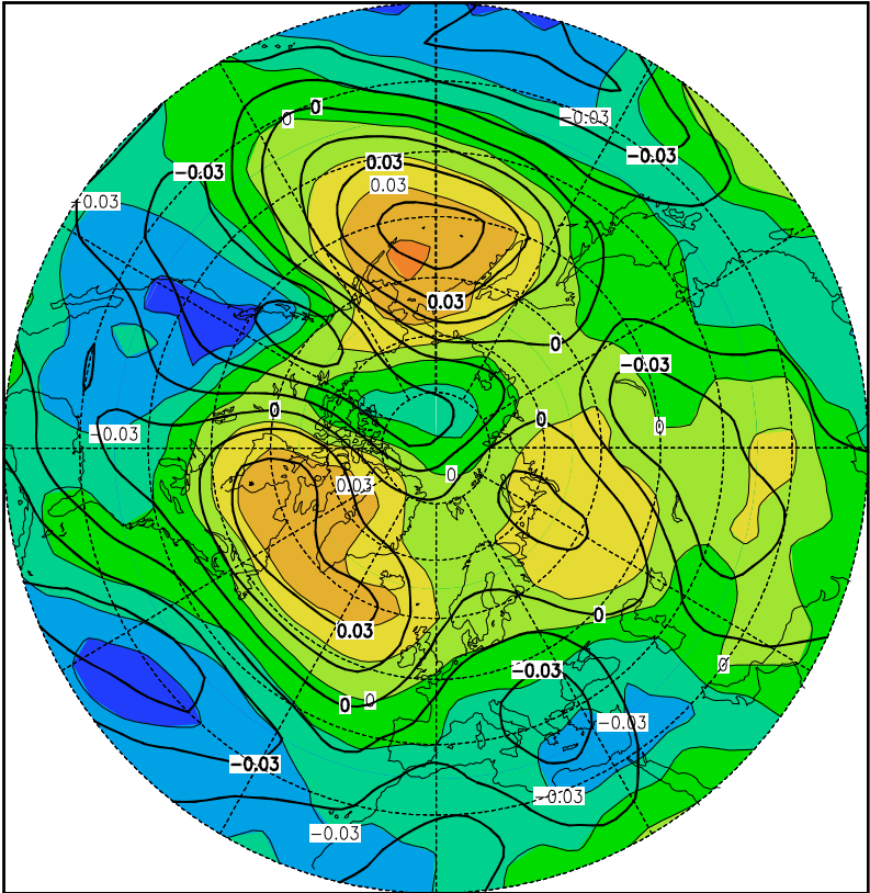
Abbildung A80: 5. Eigenvektor des Dezembers (7,2%)
