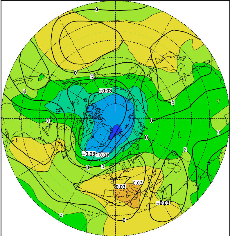
Abbildung A76: 1. Eigenvektor des Dezembers (16,9%)
