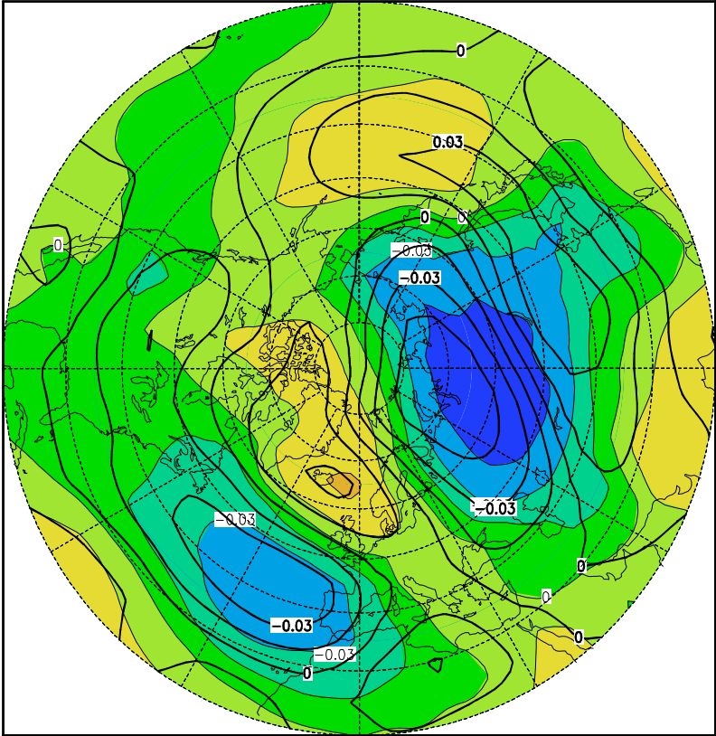
Abbildung A77: 2. Eigenvektor des Dezembers (11,1%)
