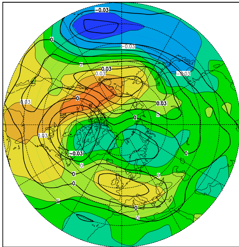
Abbildung A78: 3. Eigenvektor des Dezembers (9,7%)
