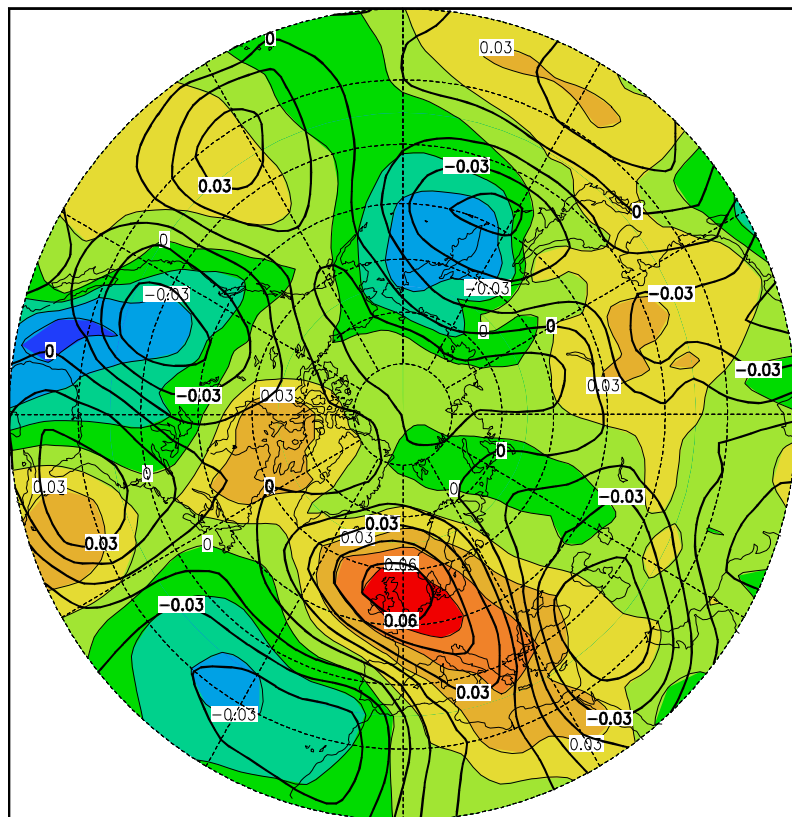
Abbildung A83: 8. Eigenvektor des Dezembers (4,0%)
