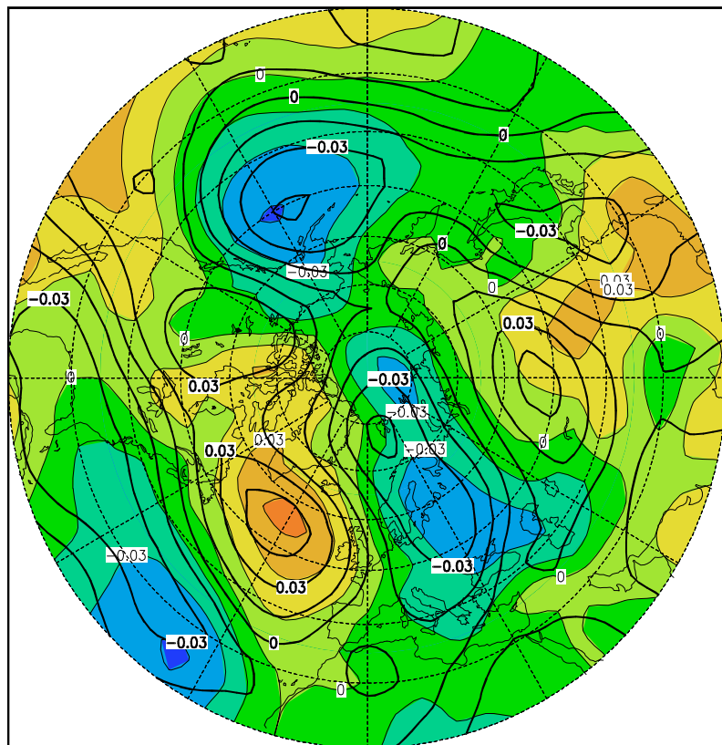
Abbildung A79: 4. Eigenvektor des Dezembers (7,6%)
