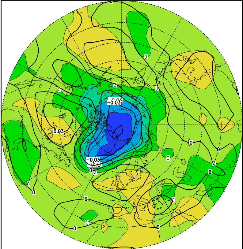
Abbildung A47: 1. Eigenvektor des Augusts (14,0%)
