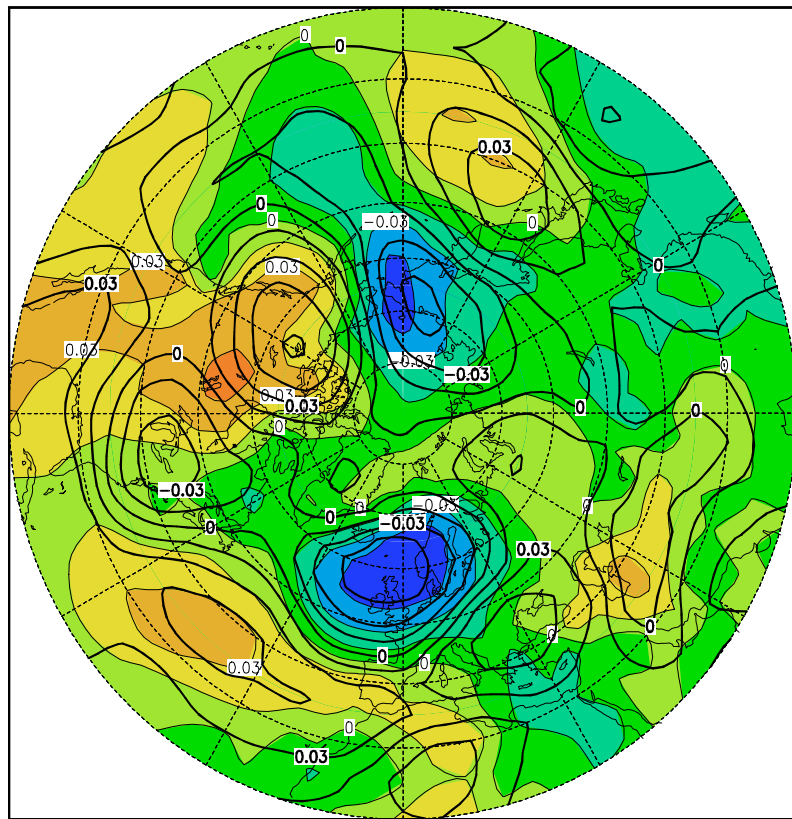
Abbildung A49: 3. Eigenvektor des Augusts (7,3%)
