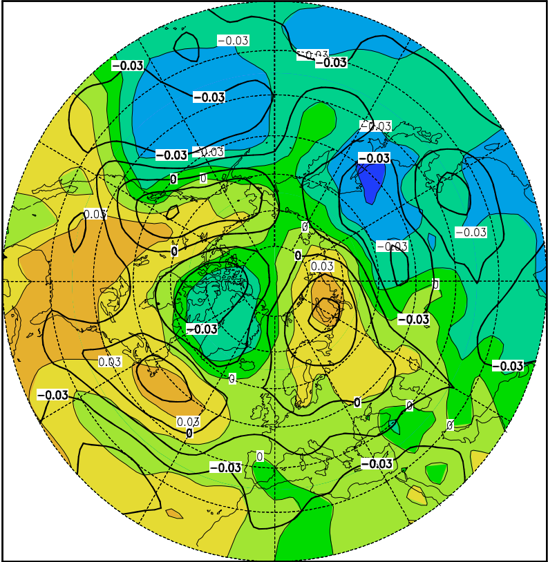
Abbildung A48: 2. Eigenvektor des Augusts (9,2%)
