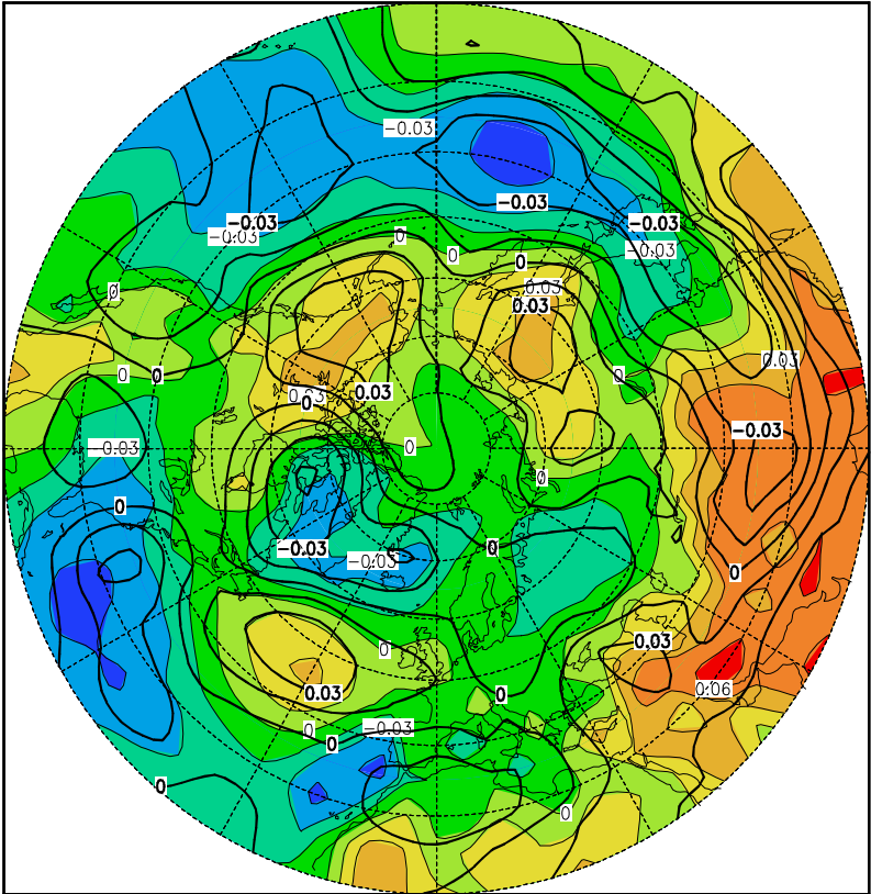
Abbildung A55: 9. Eigenvektor des Augusts (3,8%)
