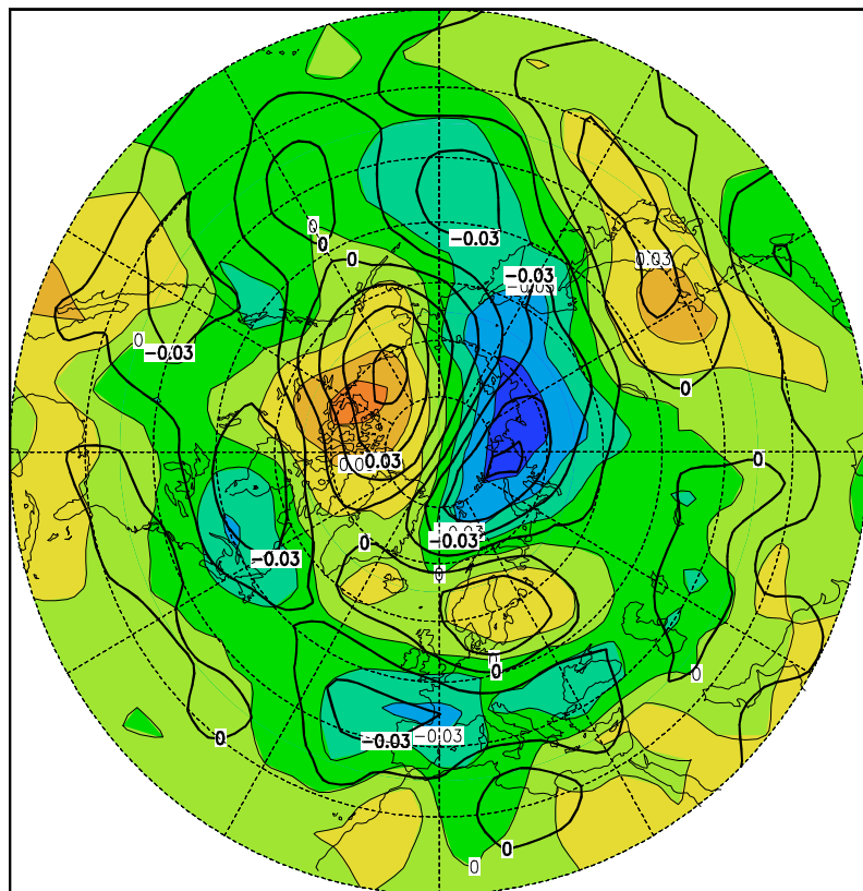
Abbildung A50: 4. Eigenvektor des Augusts (6,1%)
