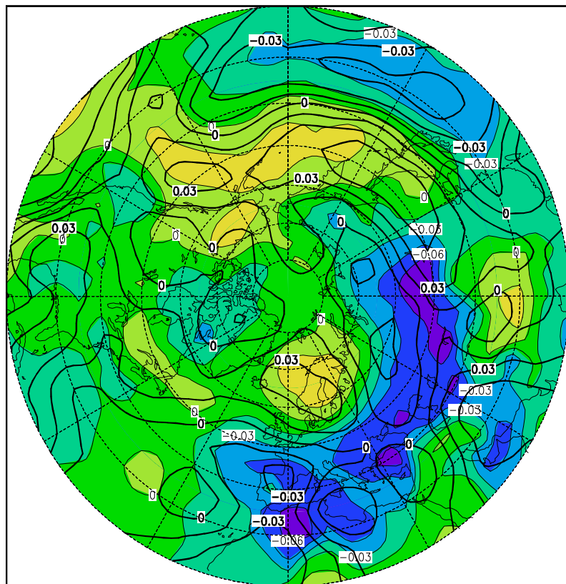
Abbildung A54: 8. Eigenvektor des Augusts (4,0%)
