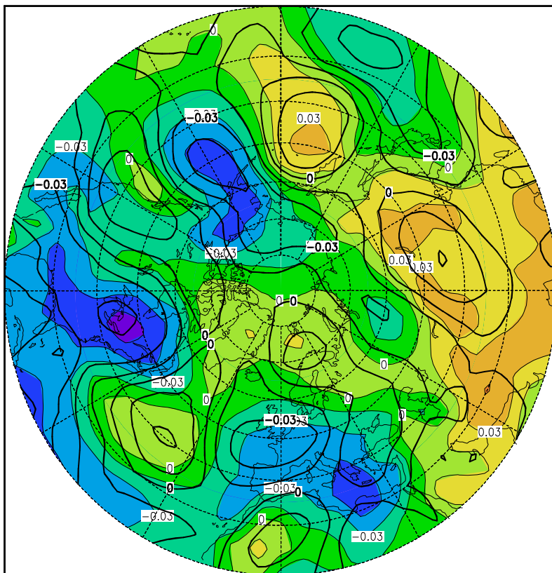
Abbildung A52: 6. Eigenvektor des Augusts (4,8%)
