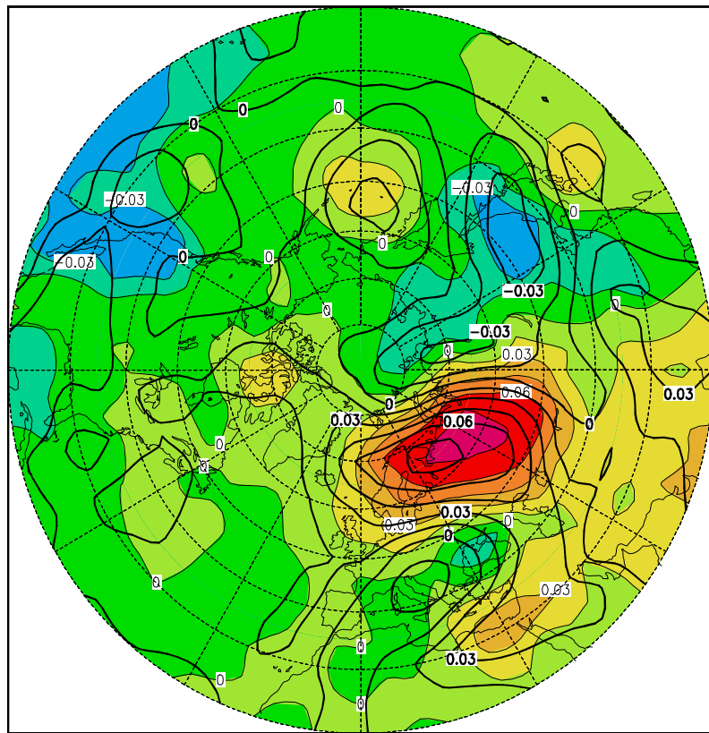
Abbildung A53: 7. Eigenvektor des Augusts (4,4%)
