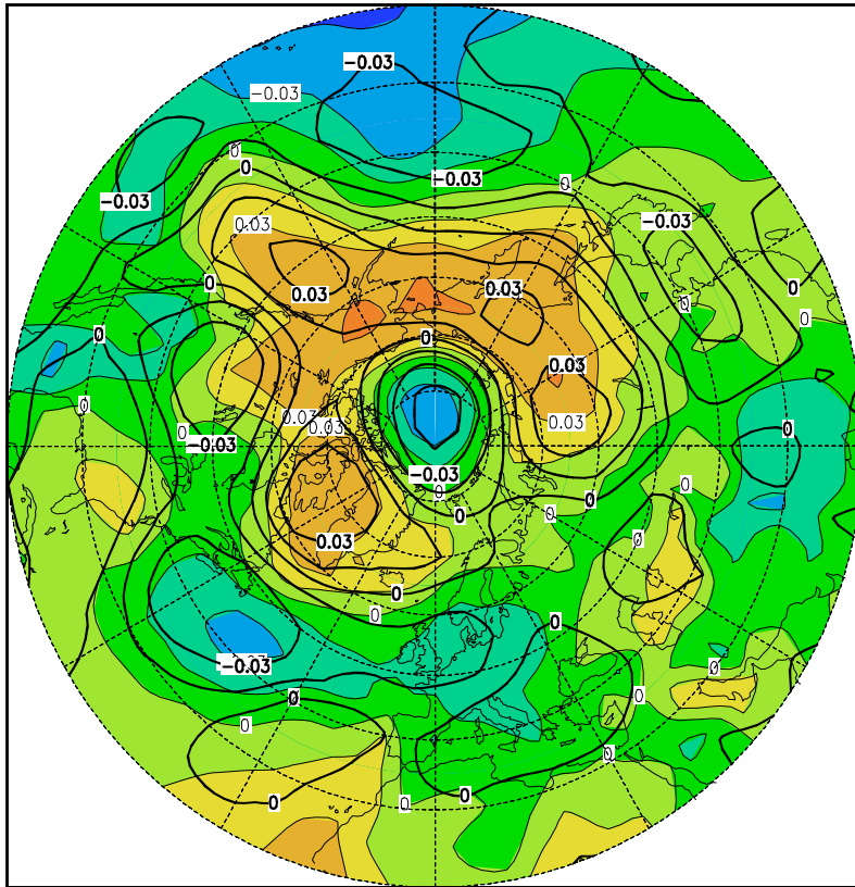
Abbildung A51: 5. Eigenvektor des Augusts (5,4%)
