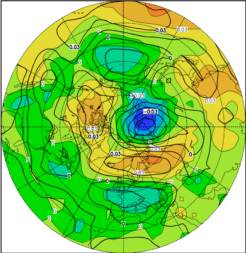
Abbildung A35: 3. Eigenvektor des Junis (6,6%)
