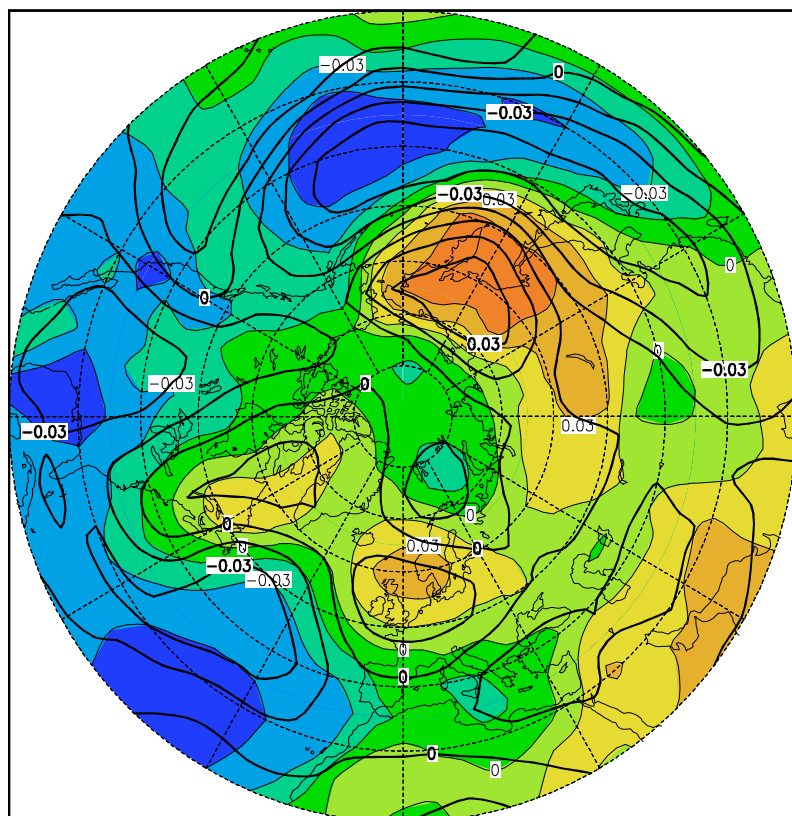
Abbildung A34: 2. Eigenvektor des Junis (9,1%)
