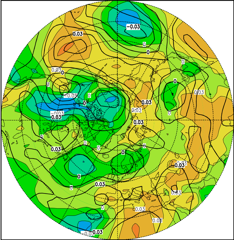
Abbildung A36: 4. Eigenvektor des Junis (6,5%)
