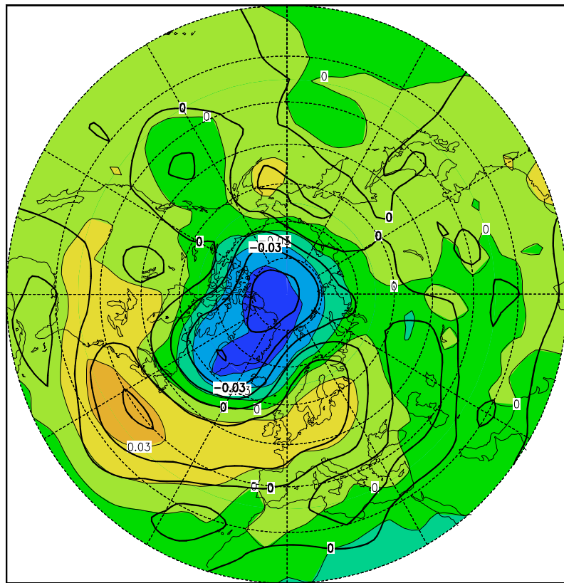
Abbildung A33: 1. Eigenvektor des Junis (15,3%)
