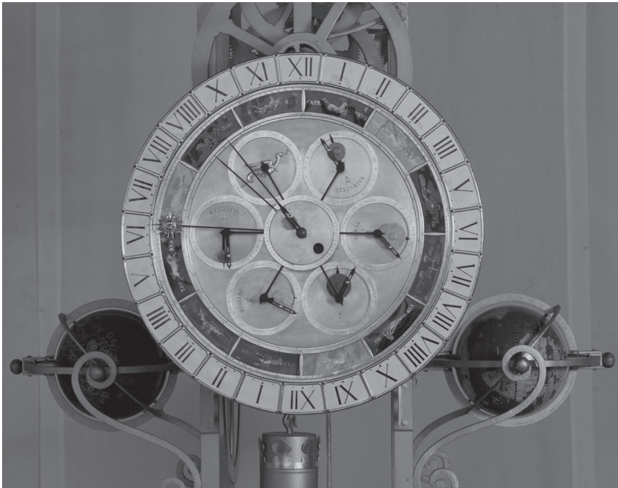
▲ Abb. 1: Lorenzo della Volpailas rekonstruiertes Planetarium im Museo della Scienza Florenz (© Museo Galileo, Florence. Photo by Franca Principe. Inventario fotografico: 41872, Orologio dei pianeti di Lorenzo della Volpaia, inv. 3817).
