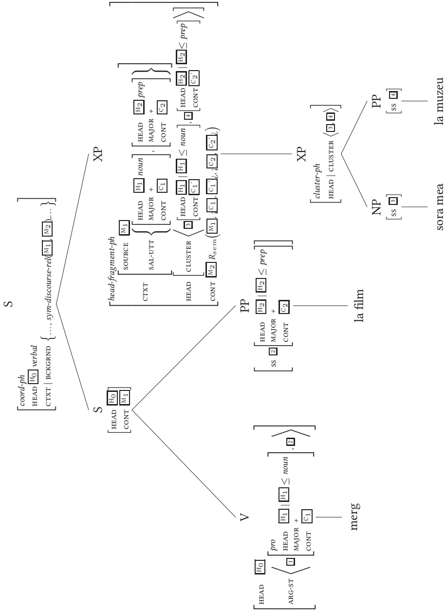
FIGURE 3.21 : Arbre simplifié de la phrase (277a)
