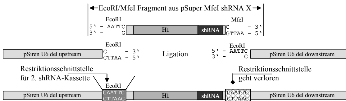
Abbildung 30: Klonierungsstrategie für multiple shRNA-Vektoren
