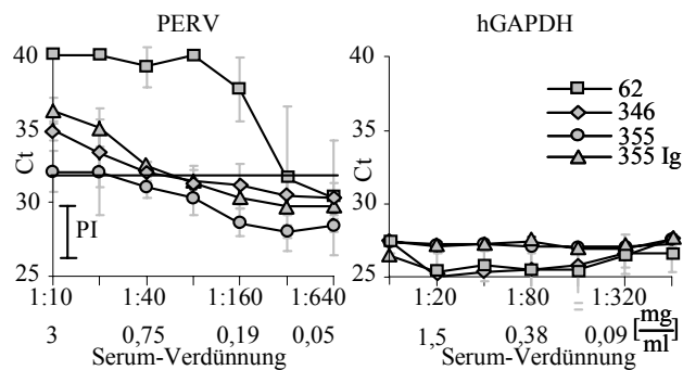
Abbildung 15: Test der Neutralisation bei Ziegen
