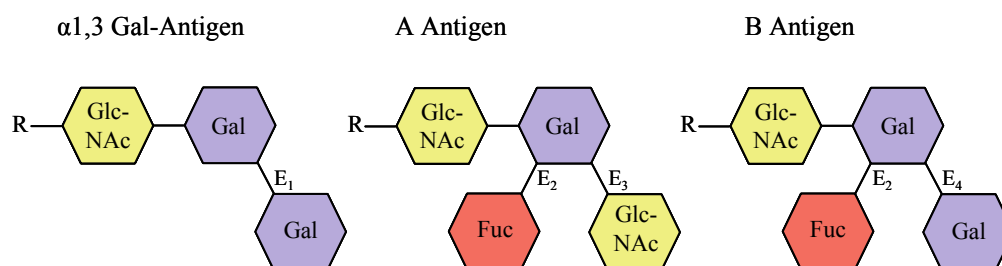
Abbildung 2: Das \alpha 1,3-Gal Epitop und die hum. Blutgruppenantigene.
