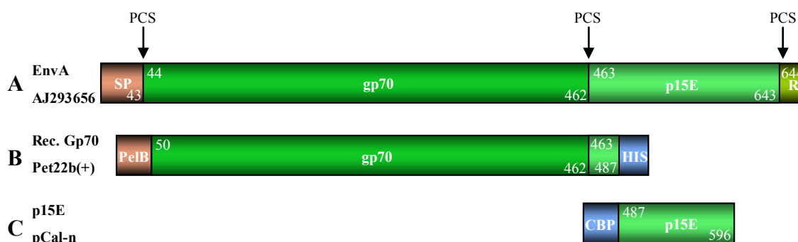
Abbildung 8: Schematische Darstellung der rekombinanten PERV-Antigene
