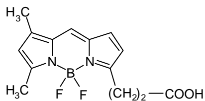
BODIPY
