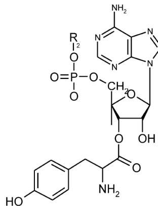
tRNA-A76
