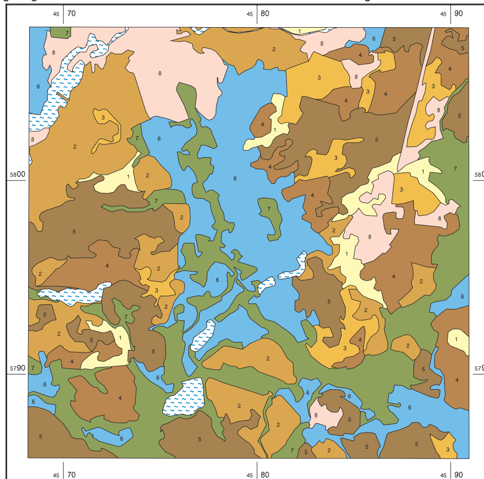
Die Bodenübersichtskarte 1 : 200 000 im Ausschnitt L3744 Potsdam, abgeleitet aus der Boden-geologischen Karte und der Flächendatenbank des Landes Brandenburg im Maßstab 1 : 50 000.
