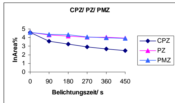
Abb.4: Halblogarithmische Auswertung der CPZ/ PZ/ PMZ Bestrahlung mit UV-A Licht
