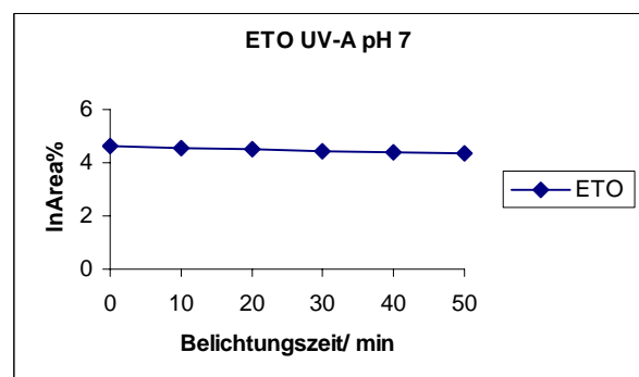
Abb.6: Halblogarithmische Auswertung der ETO Bestrahlung mit UV-A Licht
