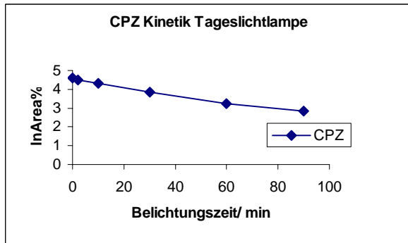
Abb.1: Halblogarithmische Auswertung der CPZ Bestrahlung mit Tageslicht
