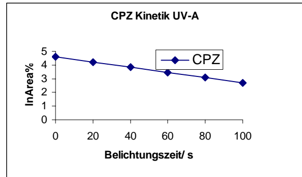
Abb.2: Halblogarithmische Auswertung der CPZ Bestrahlung mit UV-A Licht
