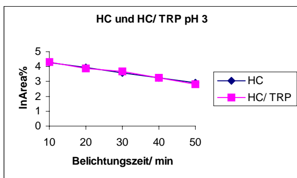
Abb.5: Halblogarithmische Auswertung der HC und HC/ TRP Bestrahlung mit UV-A Licht
