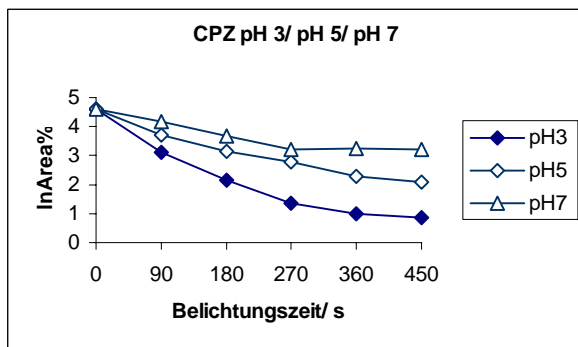
Abb.3: Halblogarithmische Auswertung der CPZ Bestrahlung bei verschiedenen pH Werten UV-A Licht
