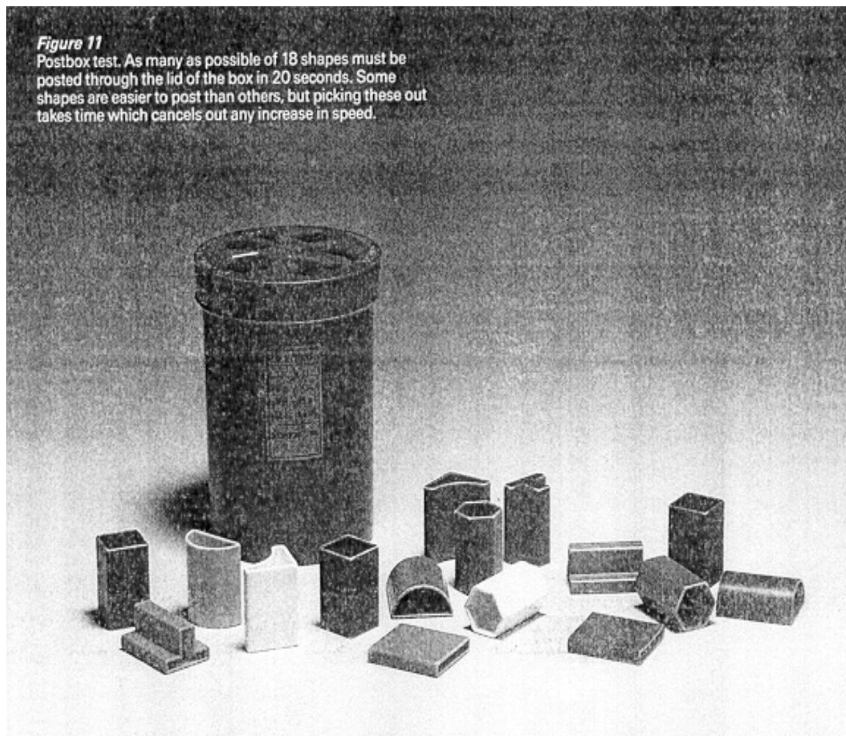
Abbildung 18: Postbox Test [140]
