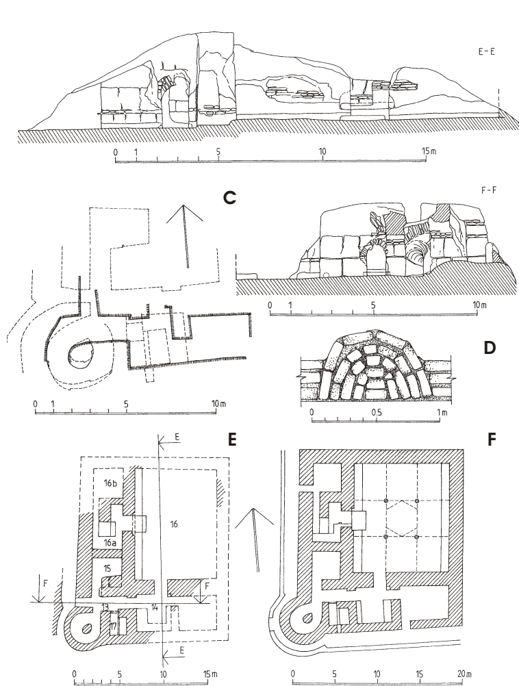
Taf. 78 Chilchudzhra (Ustrushana). Umzeichnung von N. Baimatowa (a) Räume 14 und 16. Vermessen von S. CHMELNIZKIJ. (b) Räume 13-14. Vermessen von S. CHMELNIZKIJ. (c) Rampengang. Vermessen von S. CHMELNIZKIJ. (d) Trompe in Kuppelraum 17 nach Пугачов 1975: Abb. 65. (e) Obergeschoß nach Пугачов 1975: Abb. 9. (f) Rekonstruktion des Obergeschosses nach CHMELNIZKIJ 1989: Abb. 60. (g) Querschnitt des Kuppelraums 17 ergänzt nach Пугачов 1975: Abb. 22. (h) Aufsicht auf die Kuppel von oben und unten. Darstellung von N. Baimatowa.
