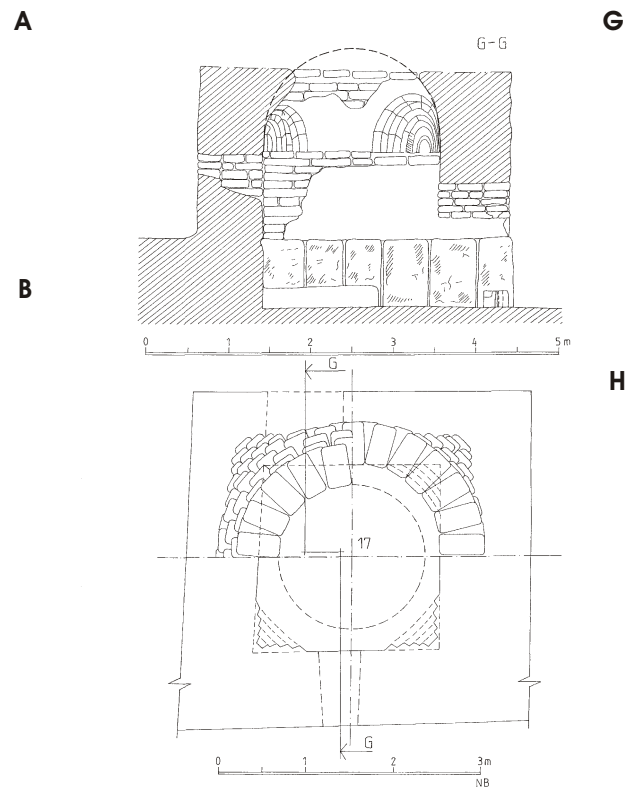
Taf. 78 Chilchudzhra (Ustrushana). Umzeichnung von N. Baimatowa (a) Räume 14 und 16. Vermessen von S. CHMELNIZKIJ. (b) Räume 13-14. Vermessen von S. CHMELNIZKIJ. (c) Rampengang. Vermessen von S. CHMELNIZKIJ. (d) Trompe in Kuppelraum 17 nach Пугачов 1975: Abb. 65. (e) Obergeschoß nach Пугачов 1975: Abb. 9. (f) Rekonstruktion des Obergeschosses nach CHMELNIZKIJ 1989: Abb. 60. (g) Querschnitt des Kuppelraums 17 ergänzt nach Пугачов 1975: Abb. 22. (h) Aufsicht auf die Kuppel von oben und unten. Darstellung von N. Baimatowa.
