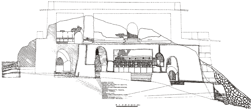
Taf. 76 Chilchudzha (Ustrushana) (a) Querschnitt zum Gesamtplan. Vermessung von S. CHMELNIZKIJ. Nach Плыатов 1975: Abb. 54. (b) Längsschnitt zum Gesamtplan. Vermessung von S. CHMELNIZKIJ. Nach Плыатов 1975: Abb. 54.
