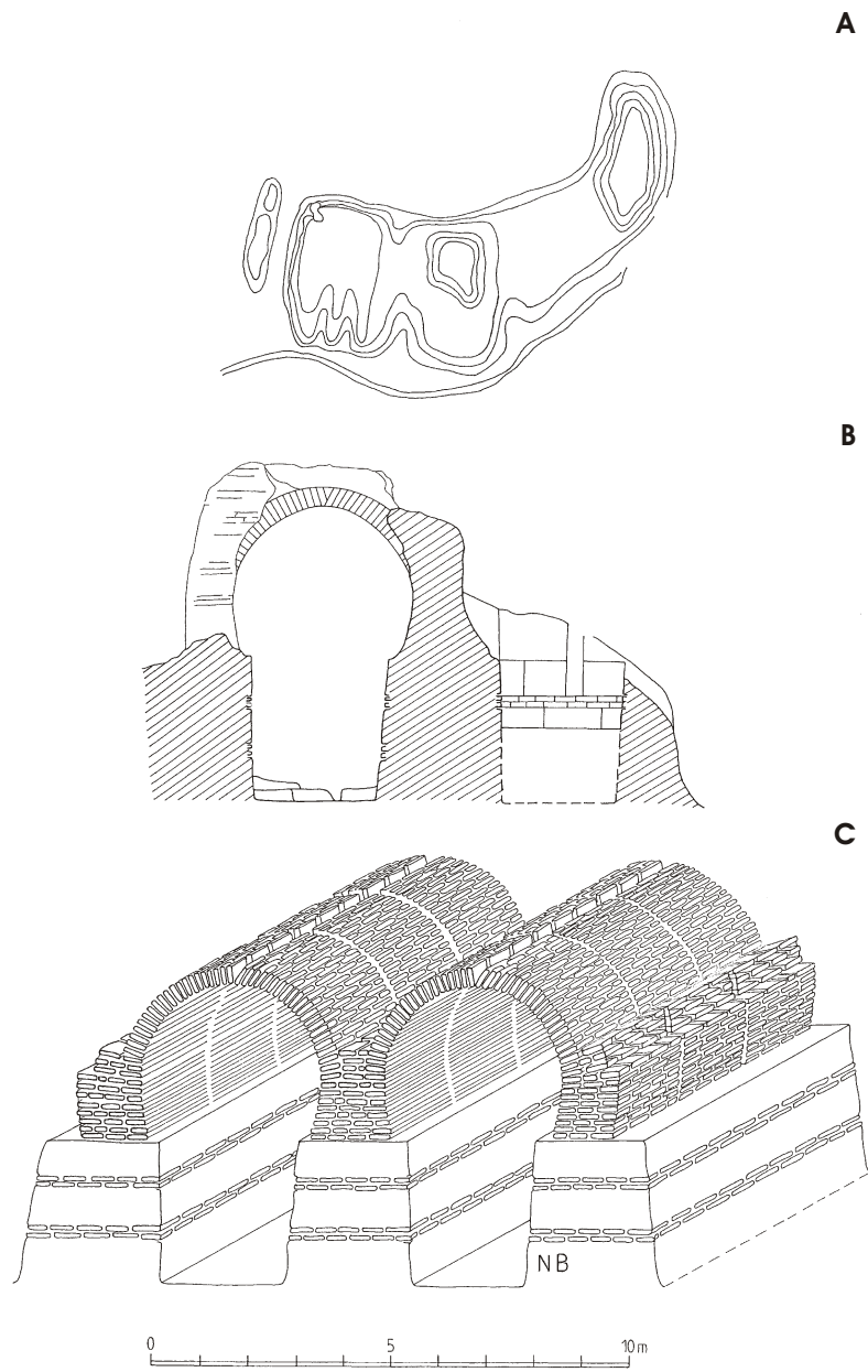
Taf. 58 Teshik Tepe (a) Lageplan des Hügels. Umgezeichnet nach Пугаченкова, Ртвеладзе 1990: 125. (b) Räume des Wohnbaus. Umgezeichnet nach Нильсен 1966: Abb. 85. (c) Isometrische Schnitt-Rekonstruktion der Räume von N. Baimatowa.
