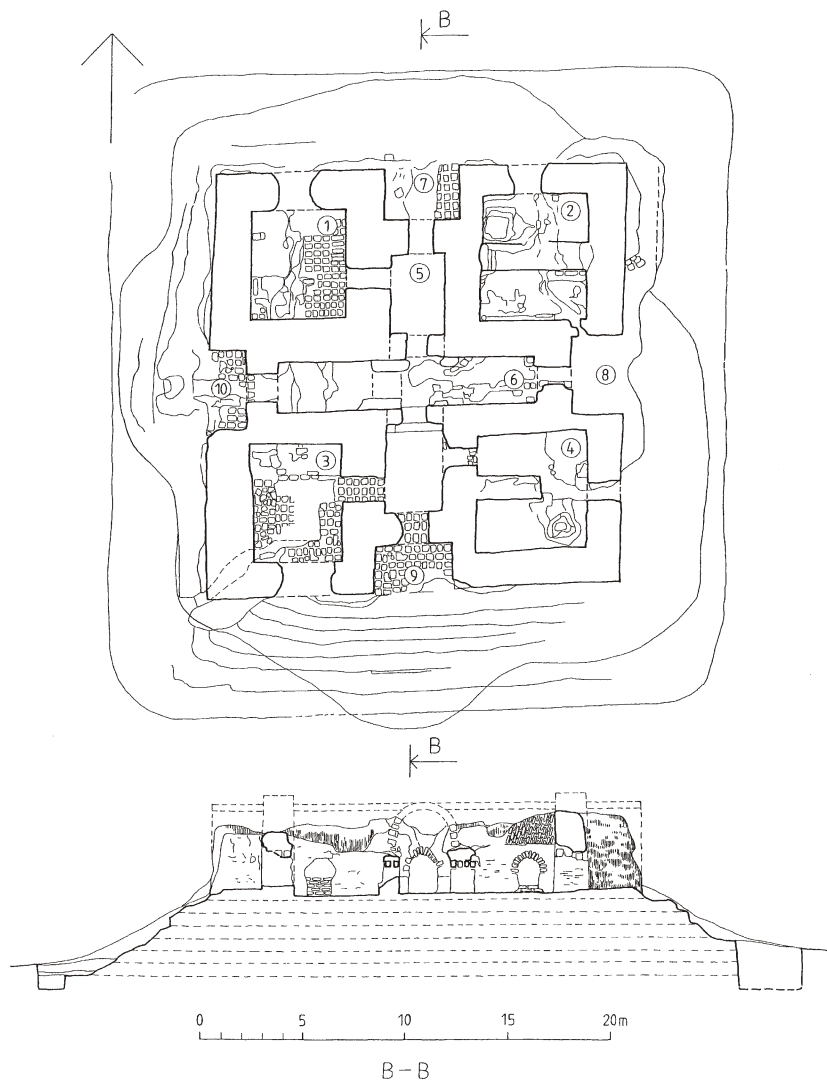
Taf. 32 Babish-Mulla-2: Baugrundriß und -Schnitt (Stand: 1962). Umgezeichnet mit eigenen Ergänzungen nach Толстов 1962: Abb. 92.
