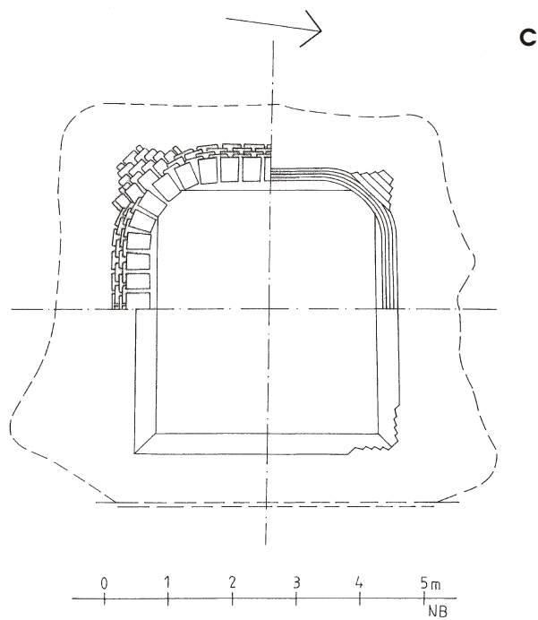
Taf. 156 Festung 36: Donjon (a) Nebenbau des Donjon. Schnitt und Grundriss umgezeichnet nach Воронина 1952: Abb. 10. (b) Nebenbau des Donjon. Schnitt und Grundriss umgezeichnet nach CHMELNIZKIJ 1989: Abb. 127. (c) Grundfläche der Kuppel über dem Nebenbau. Rekonstruktion der Ansicht von oben und unten, von N. Baimatowa.
