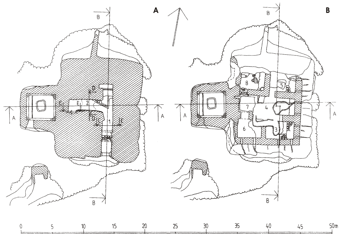
Taf. 152 Festung 36: Donjon (a-b) Erd- und Obergeschoss: Grundriss. Umgezeichnet nach Толстов 1948a: Abb. 84.
