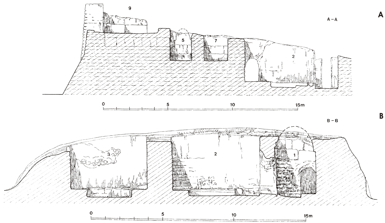
Taf. 139 Kala-i Kach-Kacha 2: Kleiner Palast (a) Querschnitt A-A. Umgezeichnet nach Негматов, Хмельницкий 1966: Abb. 28. (b) Längsschnitt B-B. Umgezeichnet nach Негматов, Хмельницкий 1966: Abb. 29.
