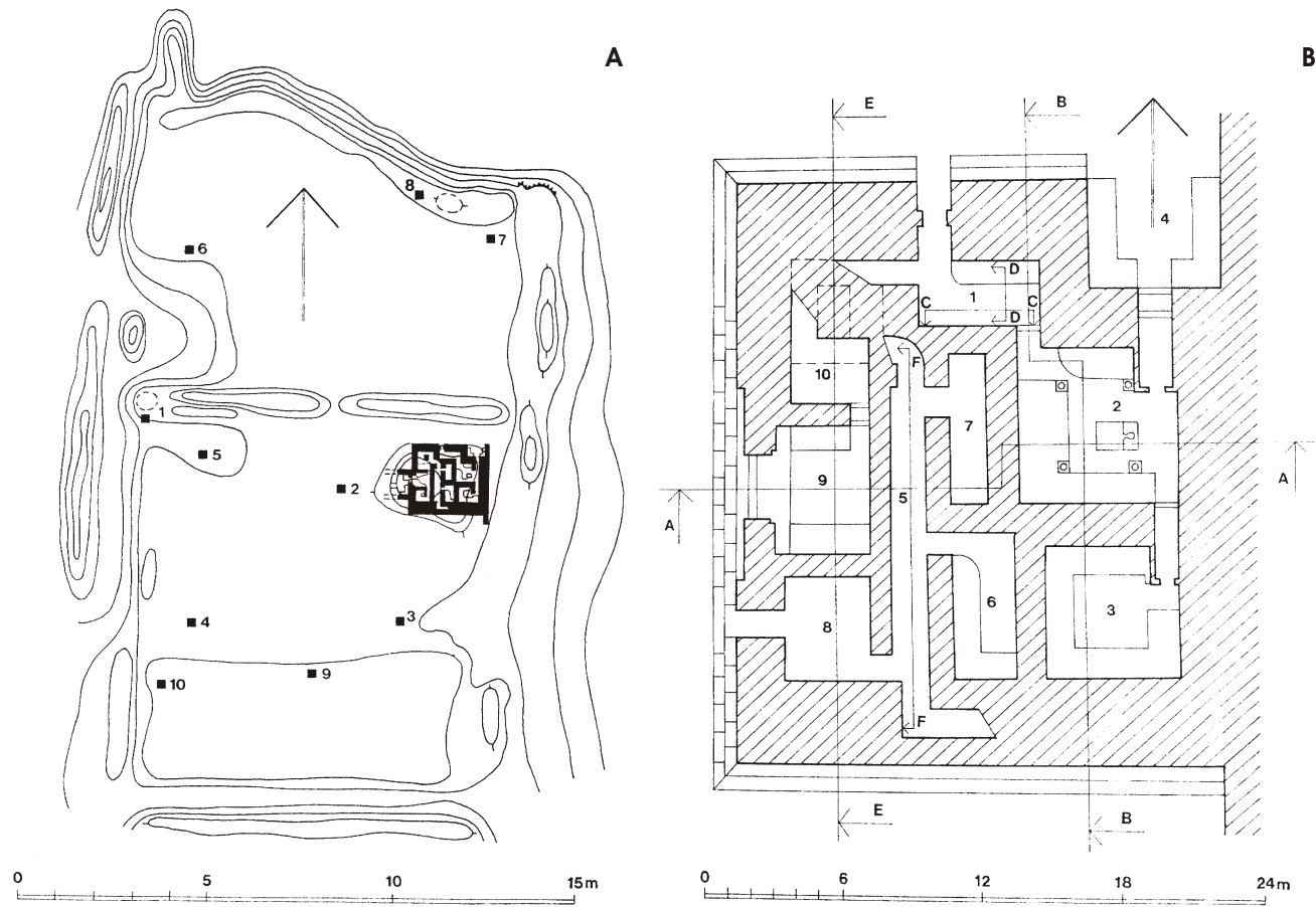
Taf. 138 Kala-i Kach-Kacha 2: Kleiner Palast (a) Lageplan der Siedlung. Umgezeichnet nach Негматов, Хмельницкий 1966: Abb. 19. (b) Grundriss des Palastes. Umgezeichnet nach Негматов, Хмельницкий 1966: Abb. 24.
