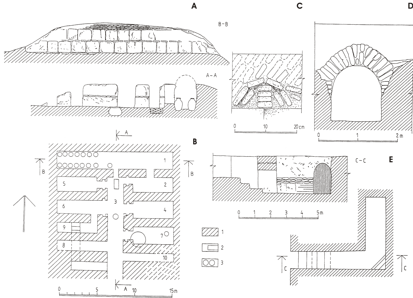
Taf. 136 Tirmizak-Tepe: Kasernenanlage (a) Quer- und Längsschnitte der Kasernenanlage. Umgezeichnet nach Германов u.a. 1973: Abb. 49. (b) Grundriss des Hauptgeschosses. Umgezeichnet nach Германов u.a. 1973: Abb. 48. Legende: 1) Mauer, 2) Sondage, 3) Vorratsbehälter. (c) Trompe im abgewinkelten Korridor. Umgezeichnet nach Германов u.a. 1973: Abb. 52. (d) Bogenzugang in den Korridor. Umgezeichnet nach Германов u.a. 1973: Abb. 52. (e) Schnitt C-C und Grundriss des abgewinkelten Korridors. Umgezeichnet nach Германов u.a. 1973: Abb. 52.
