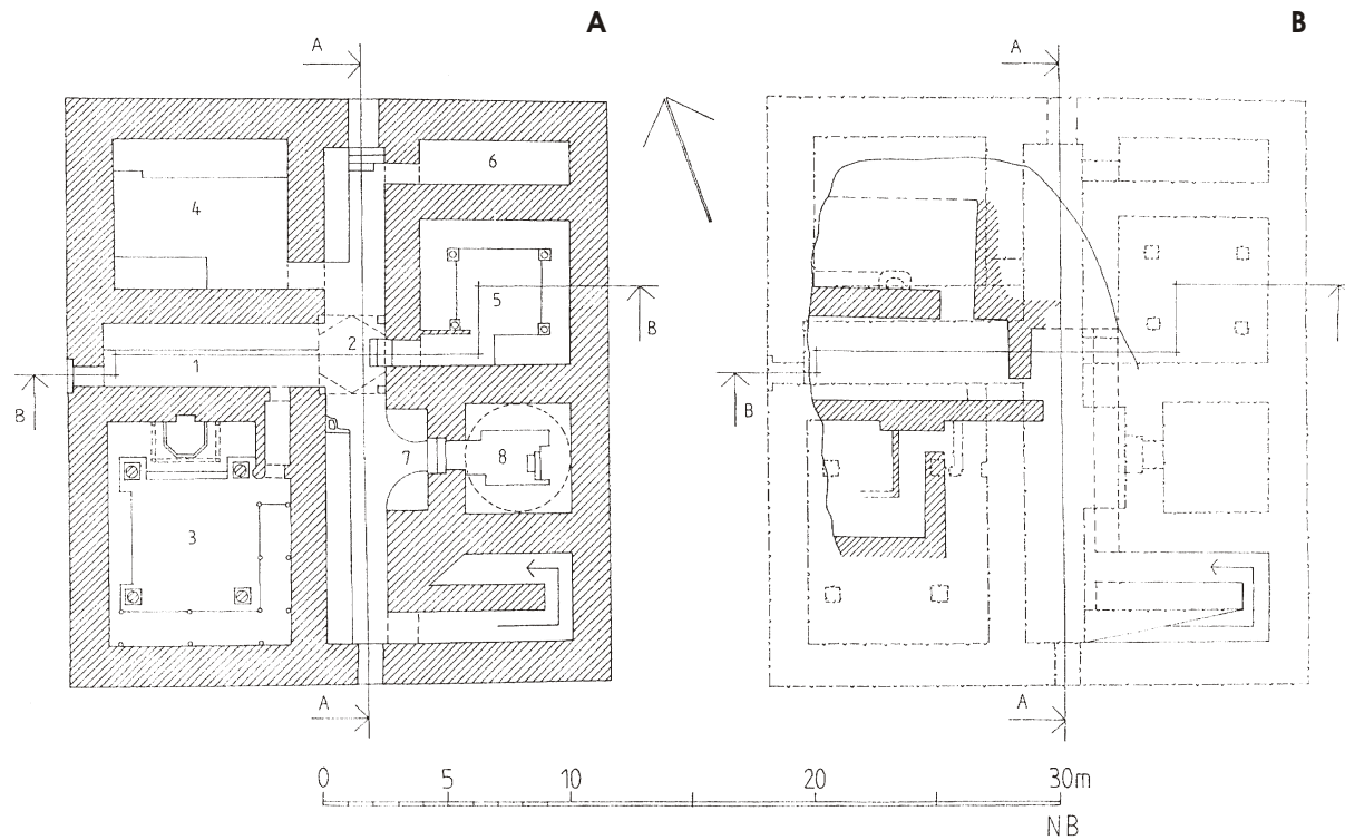
Taf. 130 Urtakurgan: Schloss (a) Grundriss des Erdgeschosses. Umgezeichnet nach HERMATOV u.a. 1973: Abb. 6. (b) Vergleichende Darstellung der Grundrisse der Erd- und Obergeschosses von N. Baimatowa. Nach HERMATOV u. a. 1973: 11, Abb. 5.
