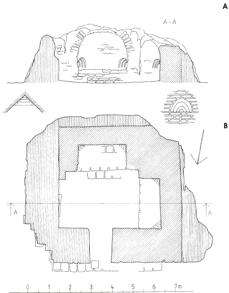
Taf. 126 Gebäude 50 (a) Längsschnitt A-A des Bauwerks. Umgezeichnet nach Неразик 1966: Abb. 44/1. (b) Grundriss des Bauwerks. Grundriss und Ansicht einer Ecktrompe. Umgezeichnet nach Неразик 1966: Abb. 44/2, 5.
