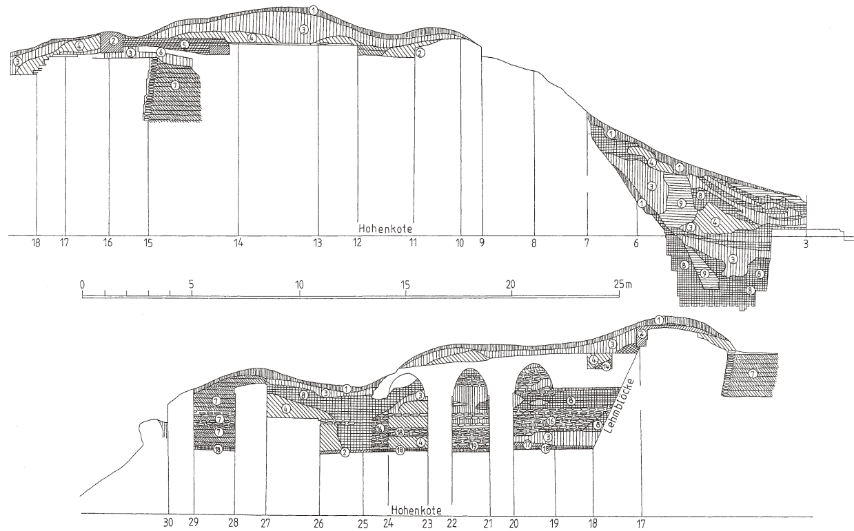
Taf. 123 Varachsha: Stratigraphischer Schnitt durch die Kaserne. Umgezeichnet nach Нильсен 1956: Abb. 7.
