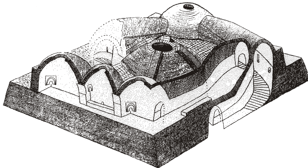
Taf. 114 Baba-ata: Isometrie des Brunnenhauses. Erste Bauperiode. Nach Areeba 1962: 130, Abb. 12.
