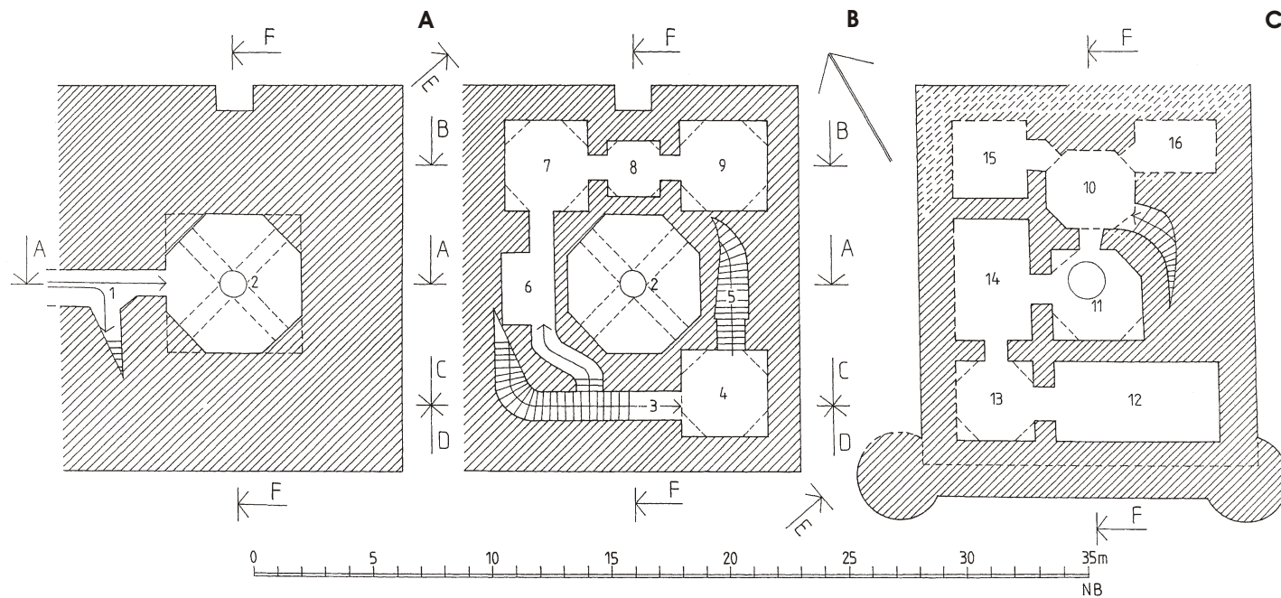
Taf. 110 Baba-ata: Grundrisse des Brunnenhauses
