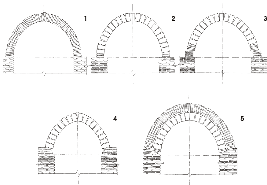
Abb. 48 Auflagerbildungen aus Lehmziegeln. Darstellung von N. Baimatowa
