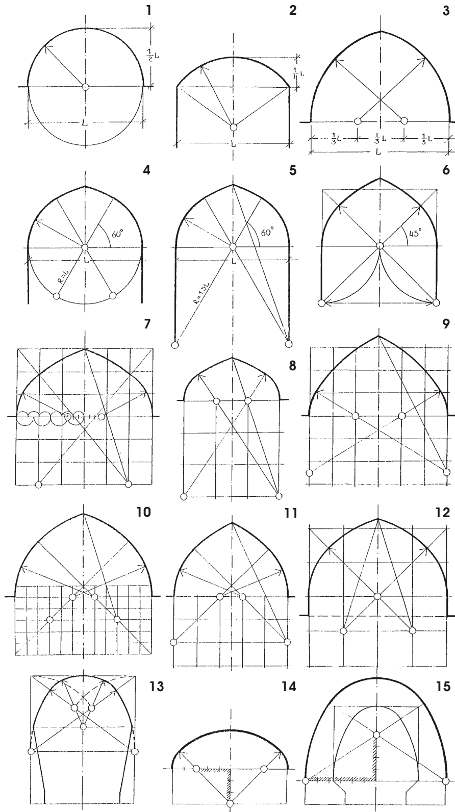
Abb. 33 Konstruktion der einfacher und komplizierter Wölbprofile in Mittelfasien Darstellung von N. Baimatowa
