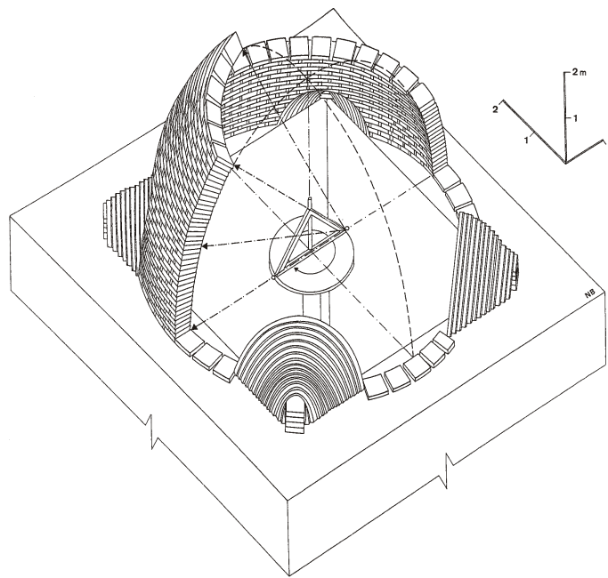
Abb. 32 Errichtung einer Kreiskuppel mit Hilfe von Seilen und hölzernen Dreieck. Darstellung von N. Baimatowa
