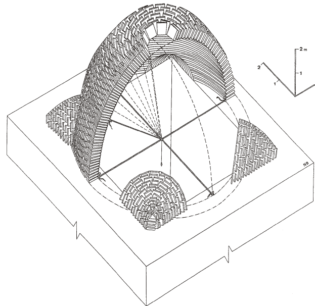
Abb. 31 Errichtung einer Kreiskuppel mit Hilfe von Seilen nach Verfahren Samarkander Baumeister. Darstellung von N. Baimatowa
