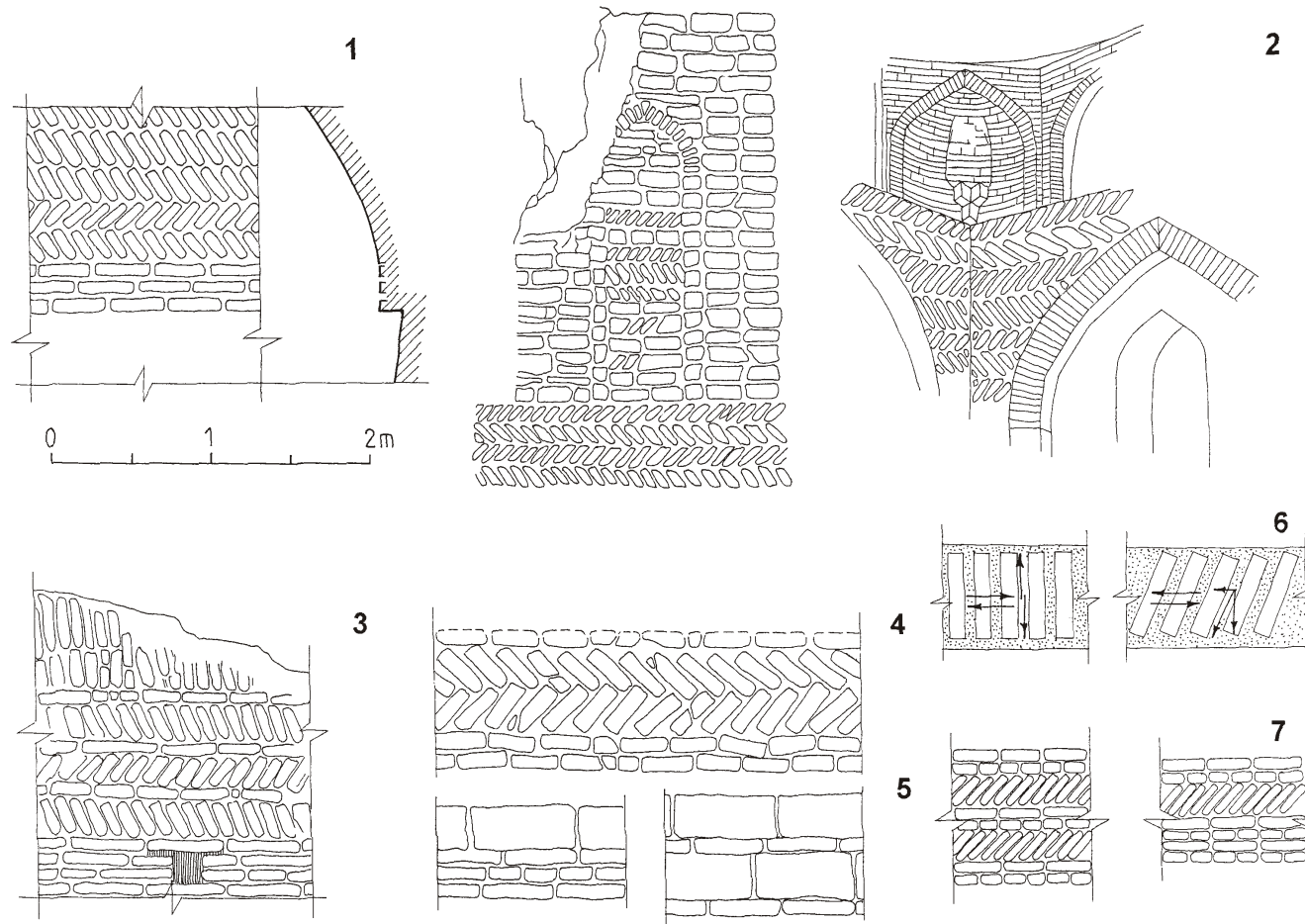
Abb. 20 Aufbau der Zäsur im unteren Teil des Tonnengewölbes:
