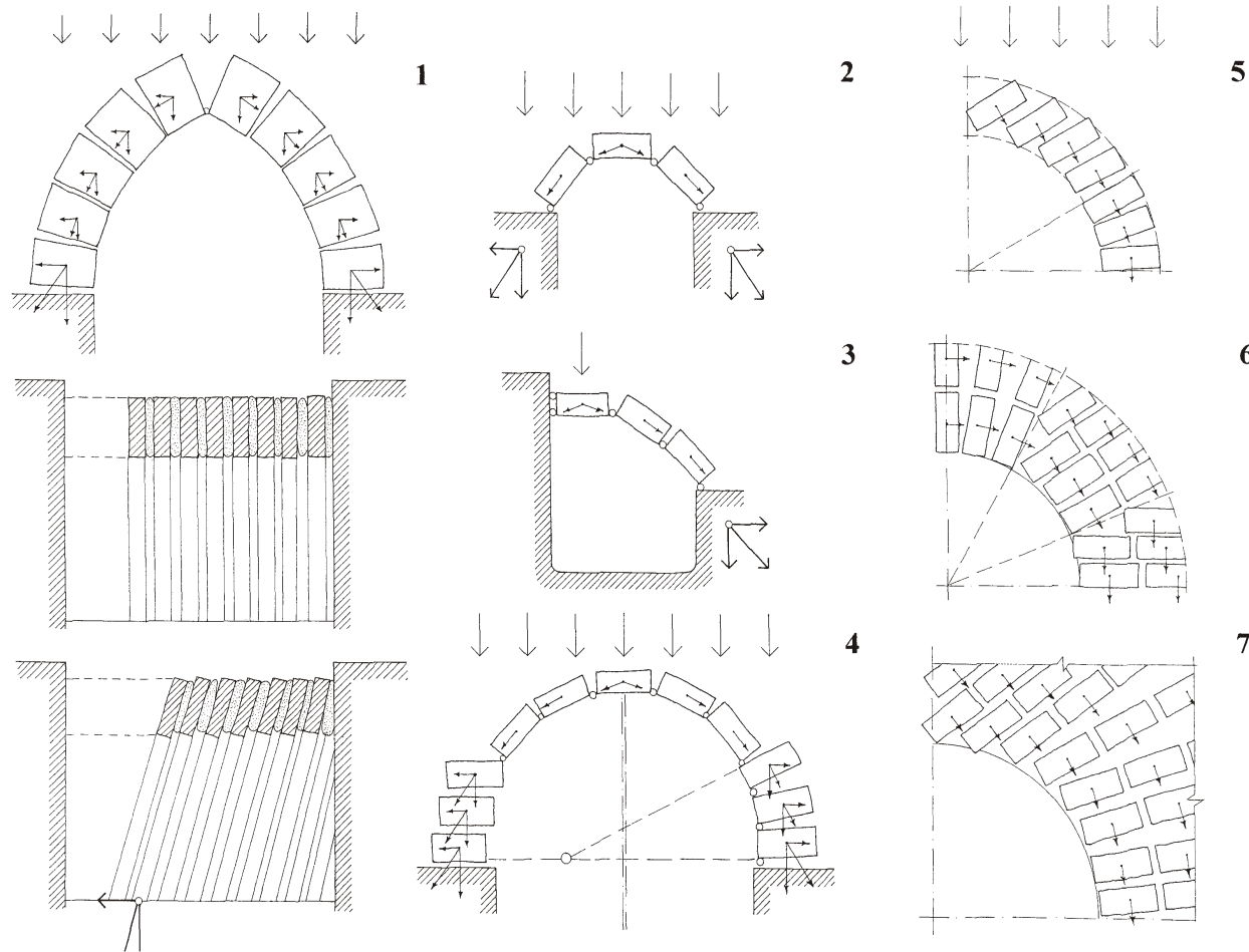
Abb. 15 Seitlicher Schub in der 1) Ringschichttonne, 2) sprengwerkförmigen Wölbung, 3) einhöftigen Wölbung, 4) Wölbung in kombinierter Ausführung, 5) Radial und angenähert radial geneigten Ziegeln in der Tonne, 6) Wölbung aus in Schichtblöcken radial geneigten Ziegel, 7) Wölbung in modifiziert-radial verlegten Ziegel
