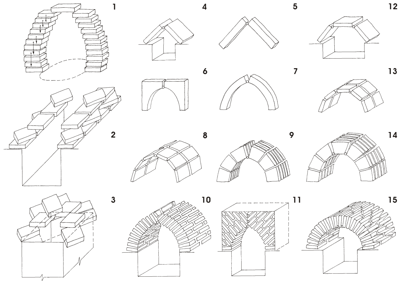
Abb. 14 Grundformen der Wölbtechnik in Mittelasien. Darstellung von N. Baimatowa
