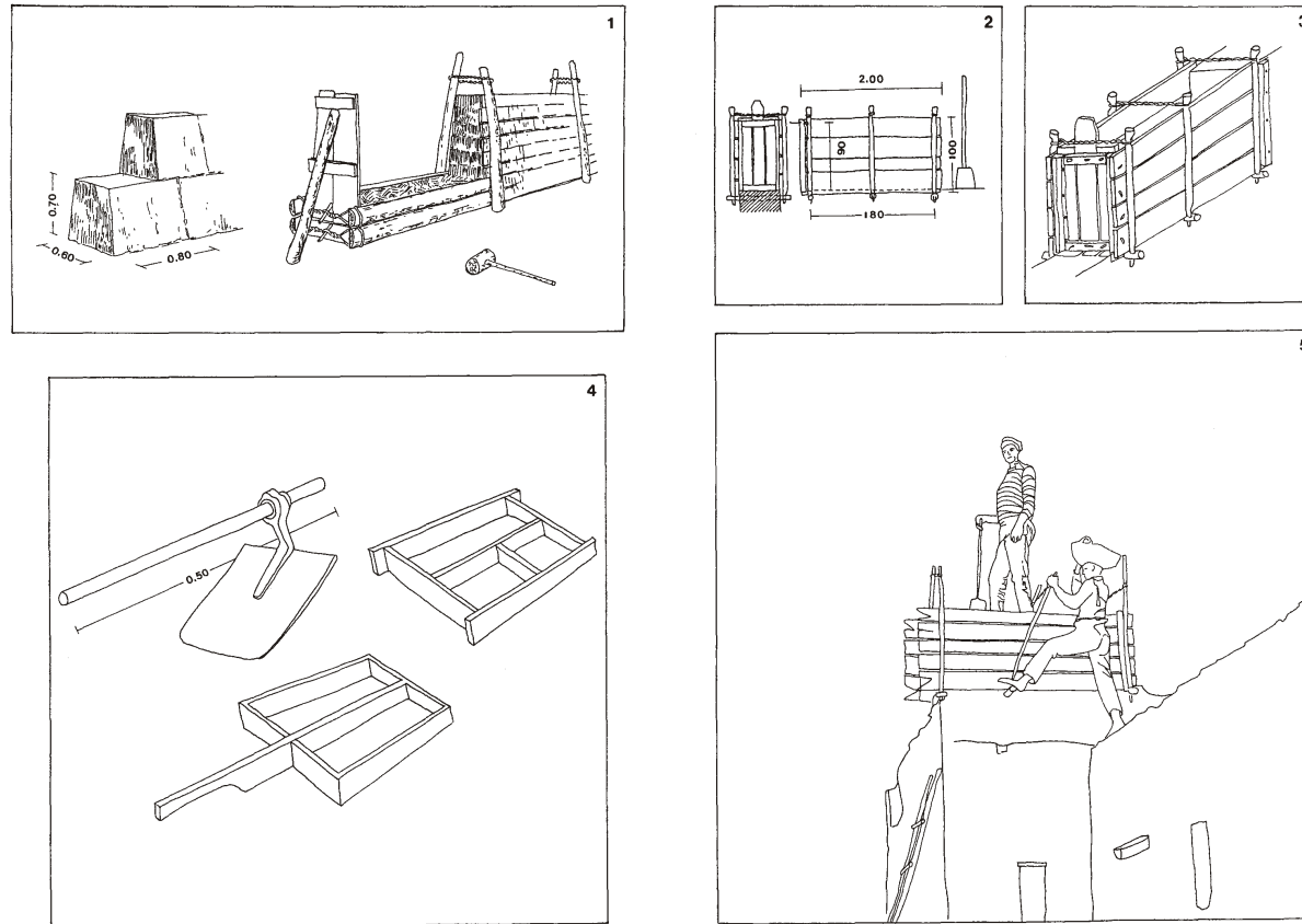
Abb. 12 Formgebung bei Lehmblöcken und Lehmziegeln.
