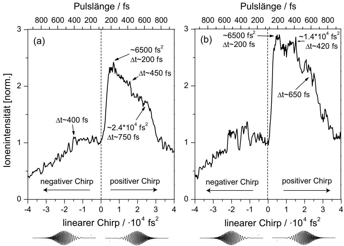
Abbildung 8.6: Abhängigkeit des Na 2 K + -Ionensignals vom linearen Chirp des fs-Pulses. (a): Das Isotop 23 Na 2 39 K. (b): Das Isotop 23 Na 2 41 K.
