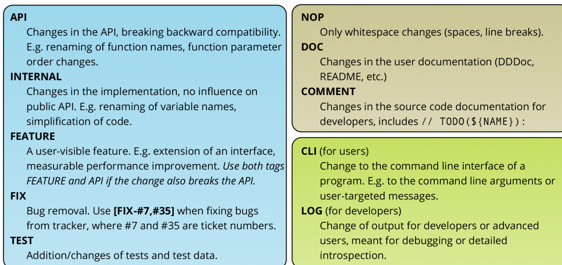
ABBILDUNG 3.6: Standardisiertes Format für Commit-Nachrichten
