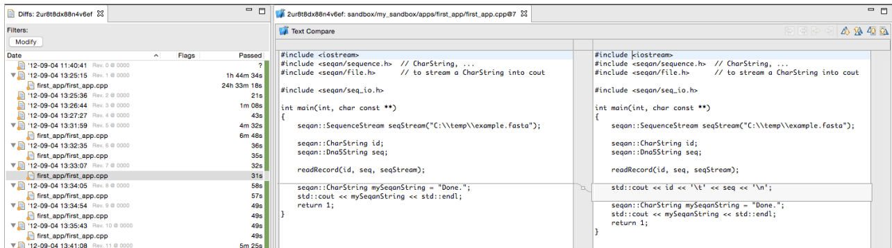
ABBILDUNG 3.18: Dieser APIUA-Bildschirmausschnitt zeigt den Probanden zur8t8dx88n4v6ef . Zu sehen sind im linken Drittel die ID des Probanden (im Tab), seine Kompilierungsversuche (Knoten erster Ordnung), alle bearbeiteten Dateien (Kindknoten), deren Kompiliererfolg (grüne, gelbe oder rote Icon-Annotation) und die auf sie verwendete Zeit.
