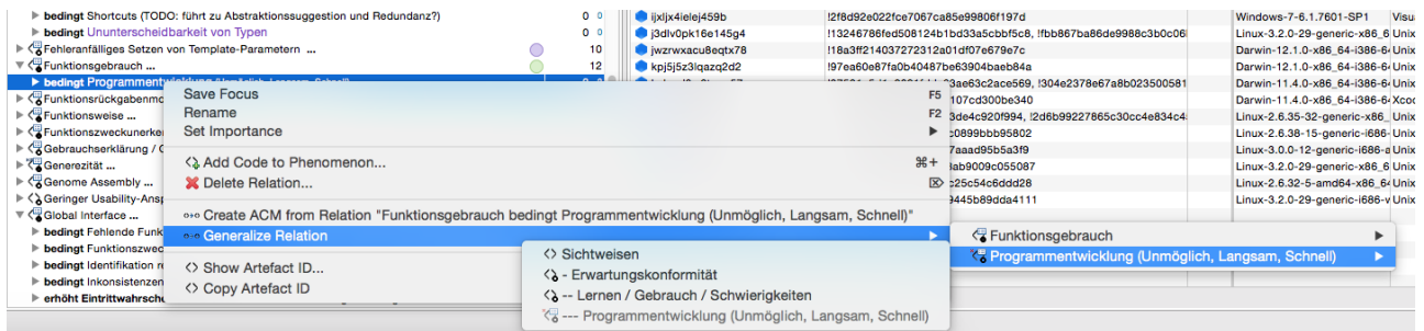
ABBILDUNG 3.20: Dieser Screenshot von APIUA zeigt die Möglichkeit zur Verallgemeinerung von Relationen.
