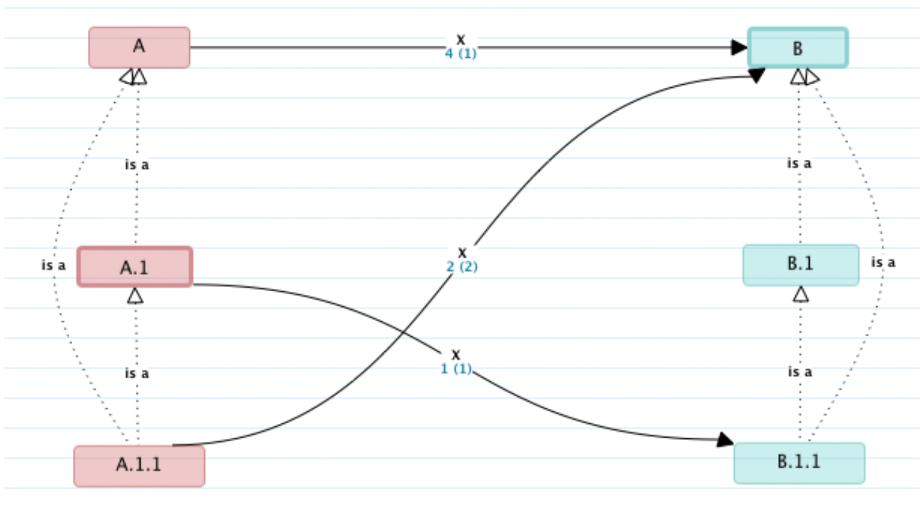
ABBILDUNG 3.35: Die Relationen \text{A.1} \vec{x} \text{B.1.1} , sowie \text{A.1.1} \vec{x} \text{B} sind implizit für \text{A} \vec{x} \text{B} . Demnach erhöht sich die Verankerung von \text{A} \vec{x} \text{B} um die Summe der Verankerungen der impliziten Relationen ( 1 + 2 = 3 ). \text{A} \vec{x} \text{B} konnte also einmal direkt und dreimal indirekt verankert werden.
