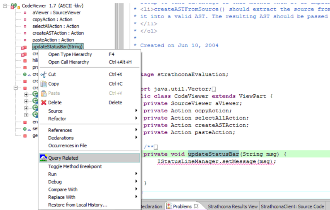
ABBILDUNG 2.21: Strathcona: Formulierung einer Beispiel-Suchanfrage (Holmes u. Murphy 2005)
