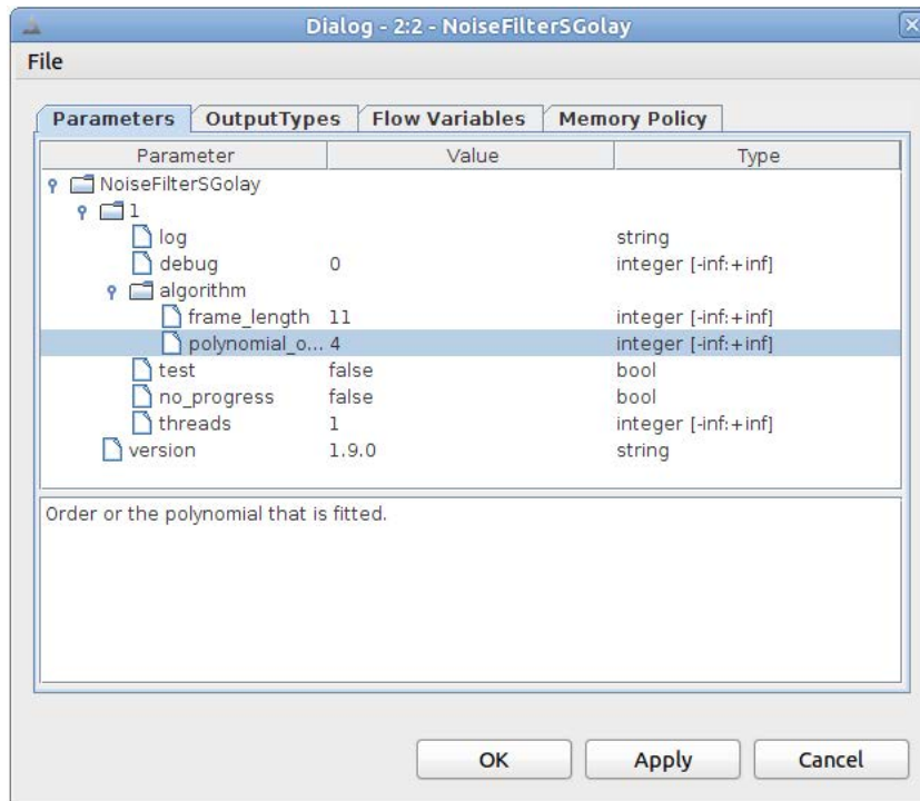
ABBILDUNG 4.5: KNIME-Konfigurationsdialog für einen CTD-basierten Knoten
