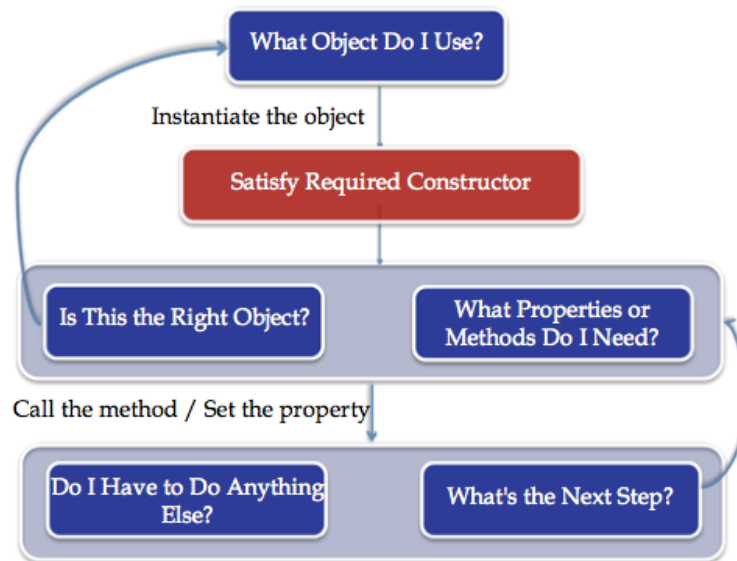
ABBILDUNG 2.11: Wenn Konstruktoren mit Parametern verwendet werden müssen und es dabei zu Problemen kommt (insbesondere IDE-Kompilierfehlern), führt dies zur Unterbrechung des Explorationsprozesses. Der API-Anwender muss den Konstruktor zunächst korrekt verwenden, bevor er fortfahren kann. (Stylos u. Clarke 2007)
