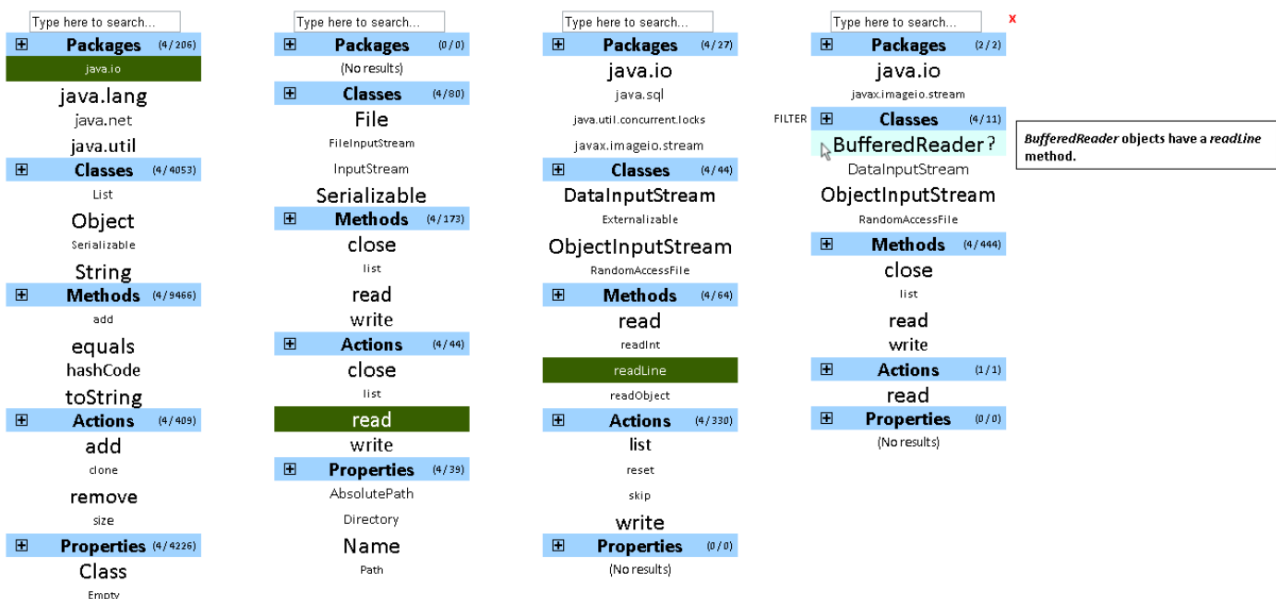
ABBILDUNG 2.18: Apatite-Dokumentationssystem (Eisenberg et al. 2010b)
