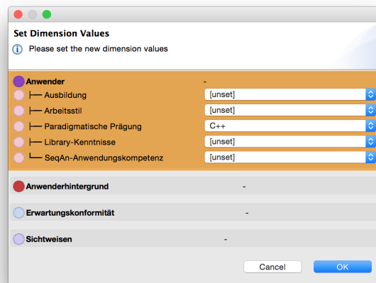
ABBILDUNG 3.20: Dieser Screenshot von APIUA zeigt die Möglichkeit zur Verallgemeinerung von Relationen.
